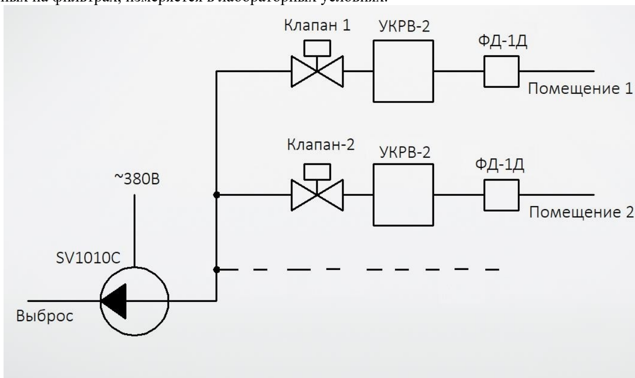
Пример линии воздухоотбора
