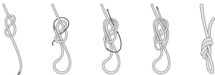
Узел «восьмерка»
