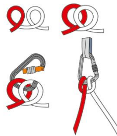
Узел «стремя»
