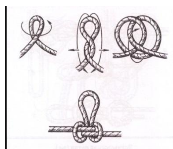
Узел «проводник»
